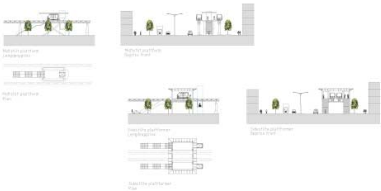
Illustrasjon 8-4: Prinsipp for holdeplasser – automatbane
