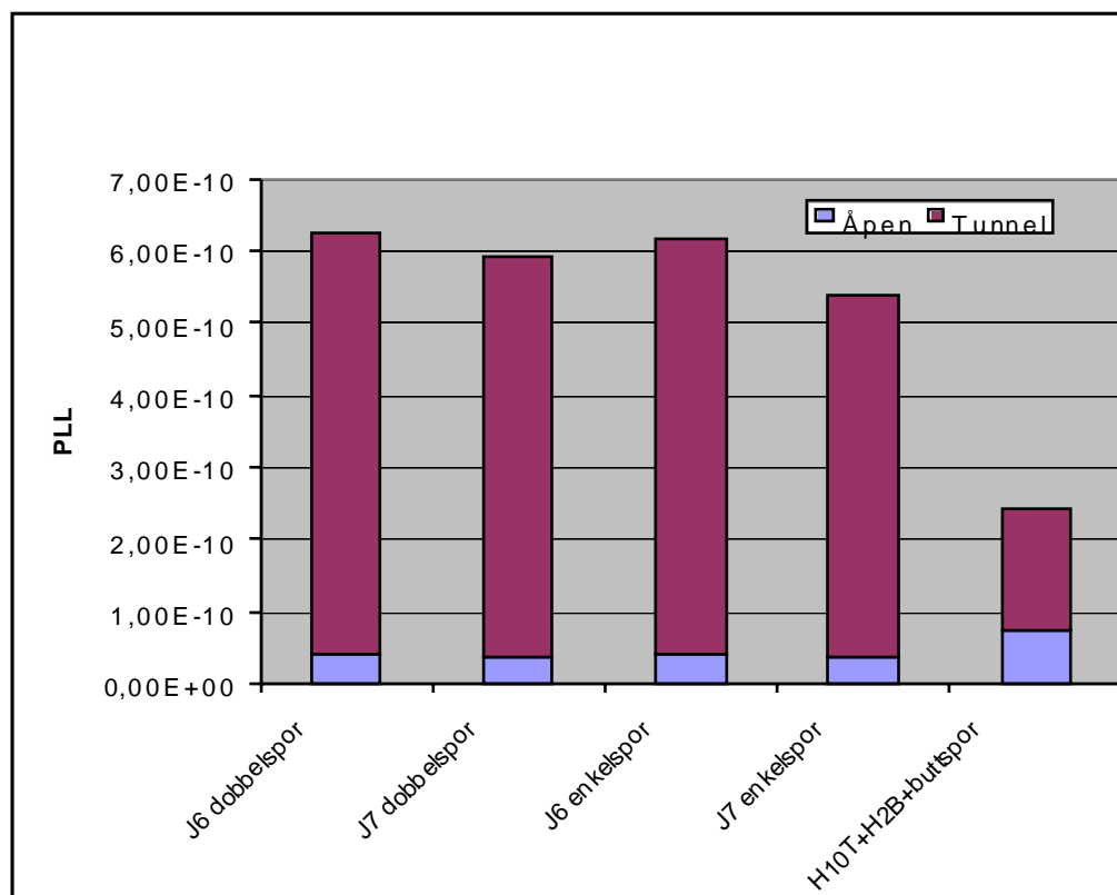
Figur 9-2: PLL per persontkilometer og år, ulike alternativer
