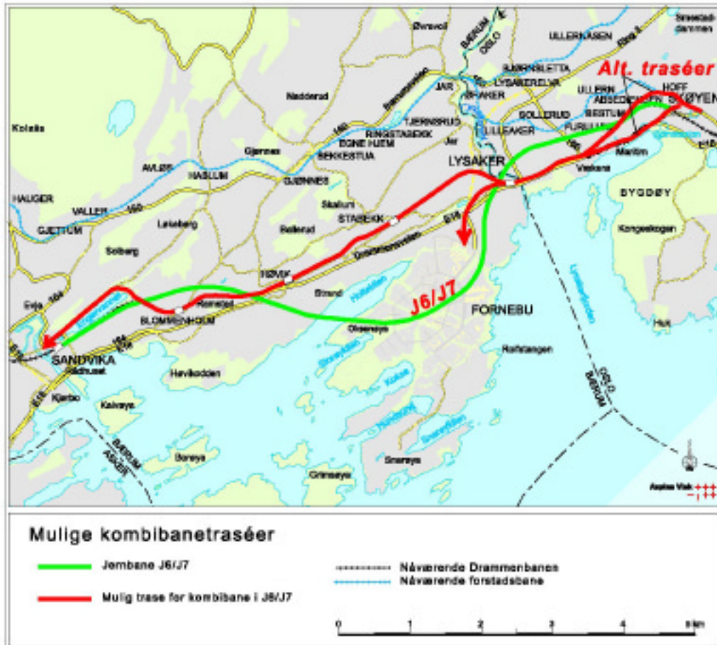
Illustrasjon 3-1: Prinsipløsning for ev. kombibanedrift i J6(J7)
