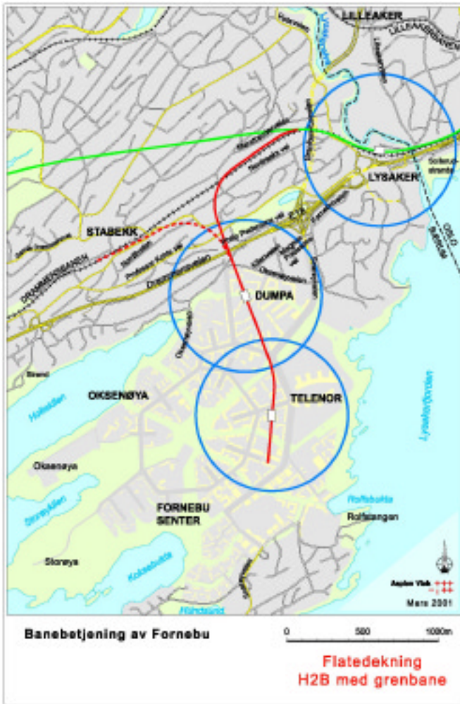
Illustrasjon 5-7: Flatedekning med tog i H2B med grenbane, områder innenfor 500 m radius fra stasjonene
